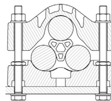
POSSIBILITÉ DE FIXATION 2: 1 X M12 FIXINGS
