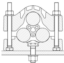
POSSIBILITÉ DE FIXATION 1: 2 X M10/M12 FIXINGS
